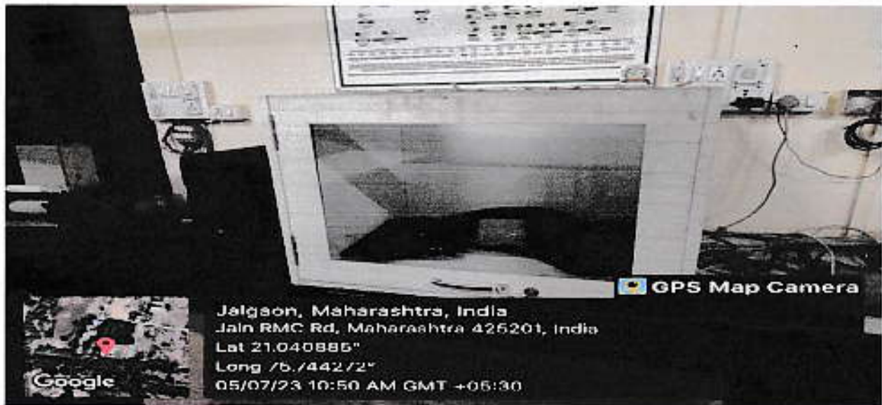
FTIR
